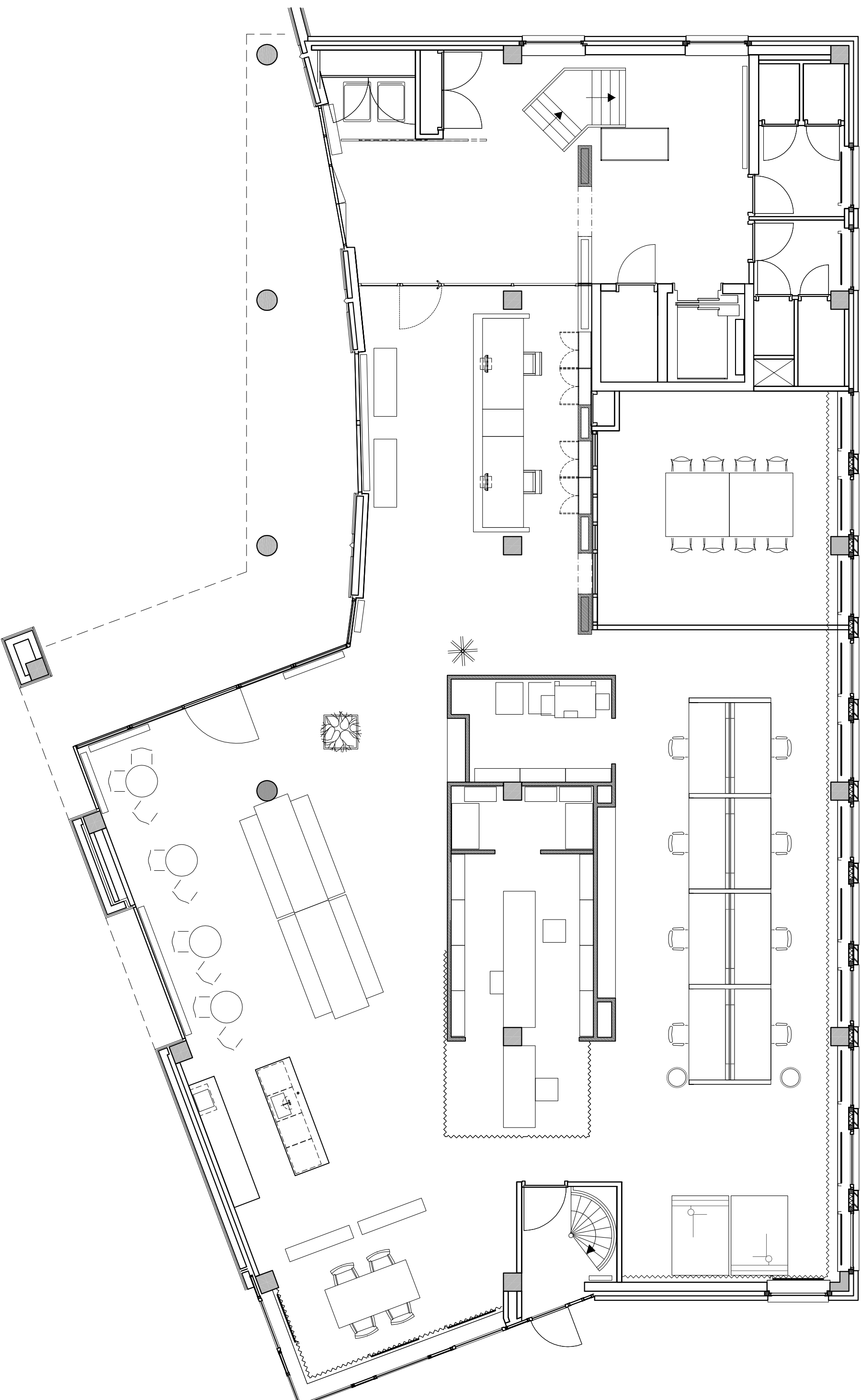
begane grond
